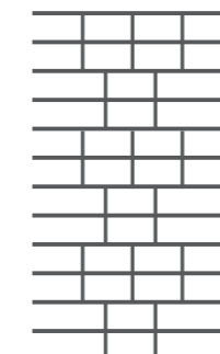
5. Szablon cegła otwarty (Stosowany w przestrzenie międzyokienne) kod: SzCO (22,5x12x18,5)x6,5x1
